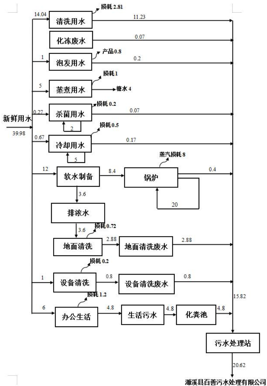
图 2-1 运营期水平衡图 \text{m}^3/\text{d}
