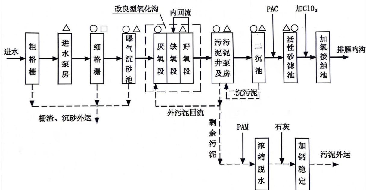
图 4.2-2 濉溪县百善污水处理有限公司处理工艺流程图
