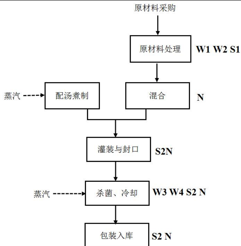
图 2-2 梨罐头食品生产工艺流程及产污节点图
