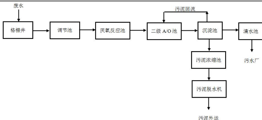
图 4.2-1 污水处理站工艺图
