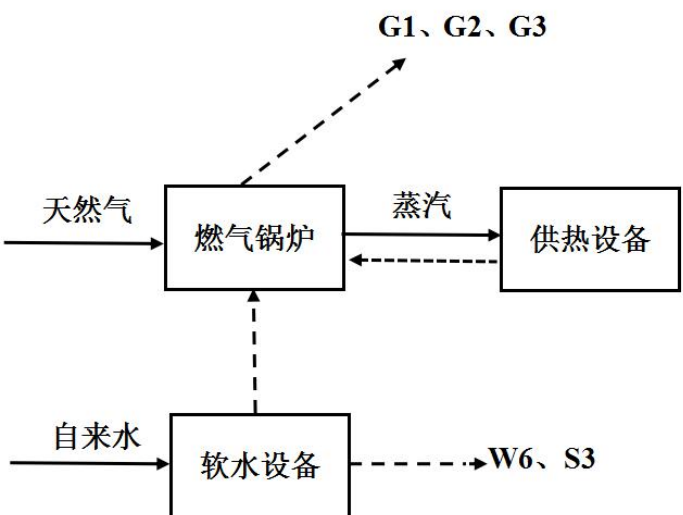
图 2-4 天然气蒸汽锅炉工艺流程图及产污环节
