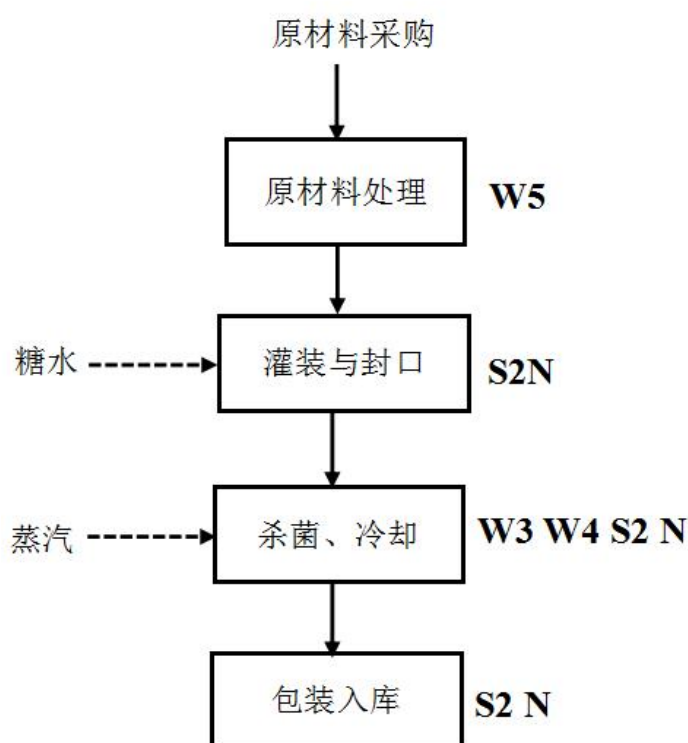
图 2-3 黄桃罐头食品生产工艺流程及产污节点图
