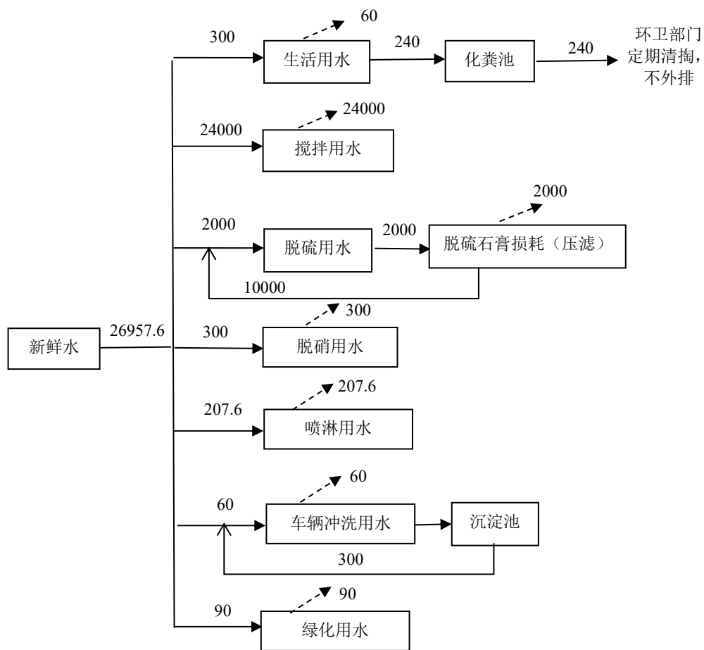
图2-1技改后全厂水平衡图 (t/a)
