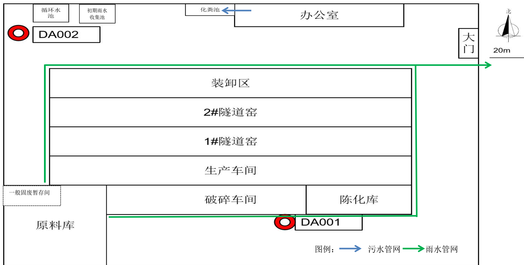
附图 3 项目雨污管网分布图
