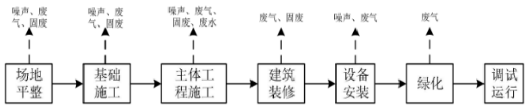
图 2-2 项目施工期工艺流程及产污环节示意图
