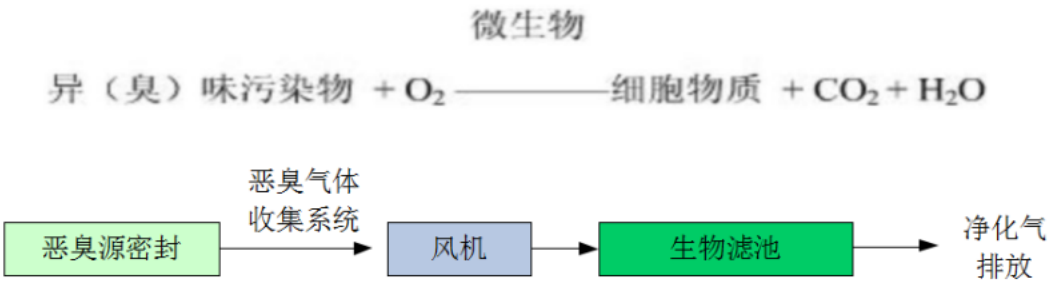
图 4-1 生物滤池除臭系统工艺流程图
