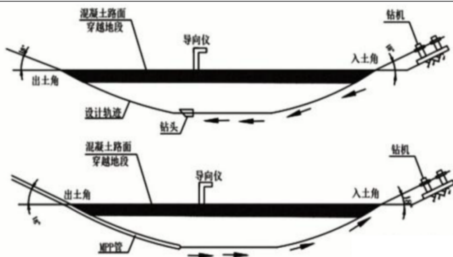
图 2-4 拉管法施工工艺图
