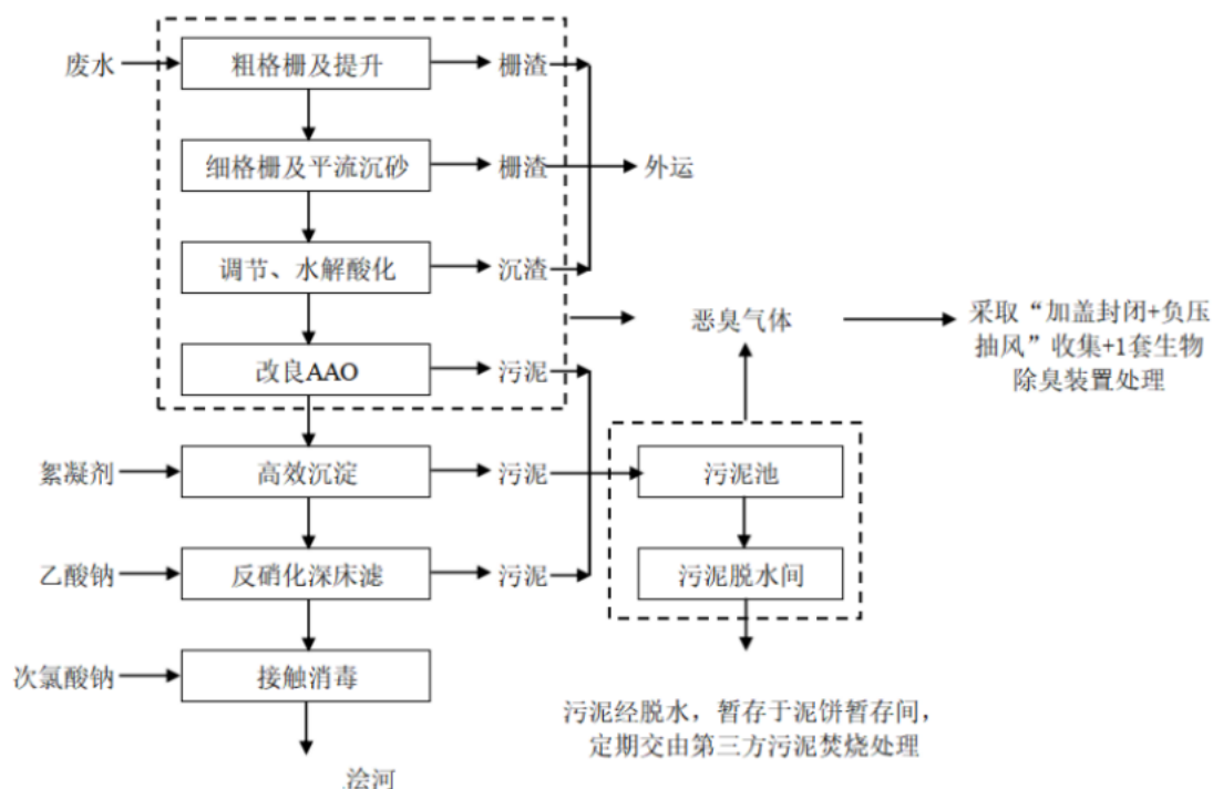
图 2-5 污水处理厂生产工艺流程及产污环节图
