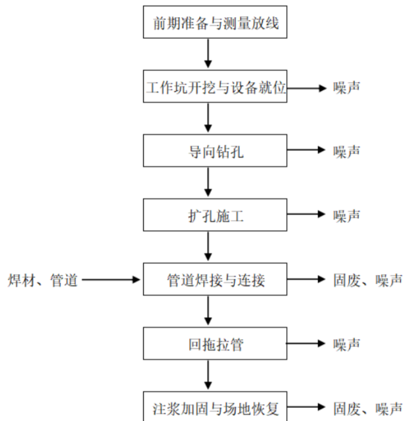
图 2-3 新建管网工程工艺流程及产排污节点图
