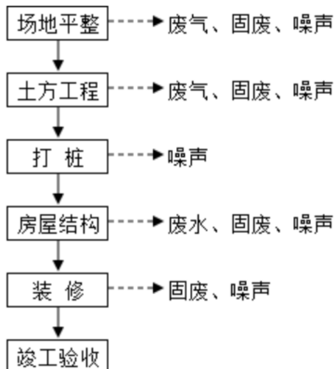
图 2-2 项目施工期工艺流程及产污环节示意图
